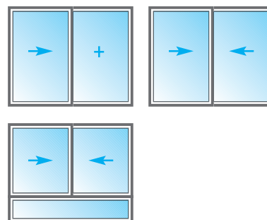
Largeur max. avec 2 vantaux: 3500 mm
